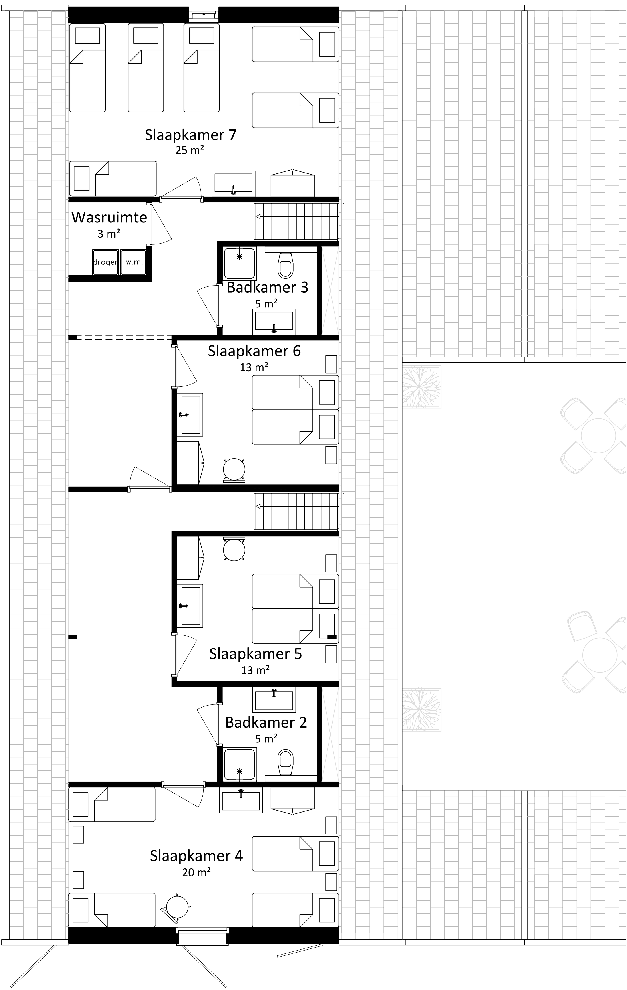
1e verdieping
